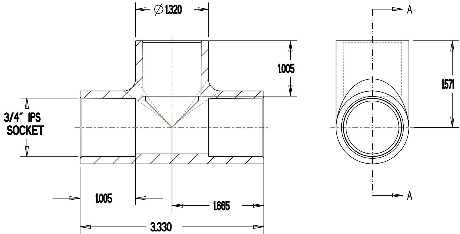
SECTION A-A SCALE 1.000
