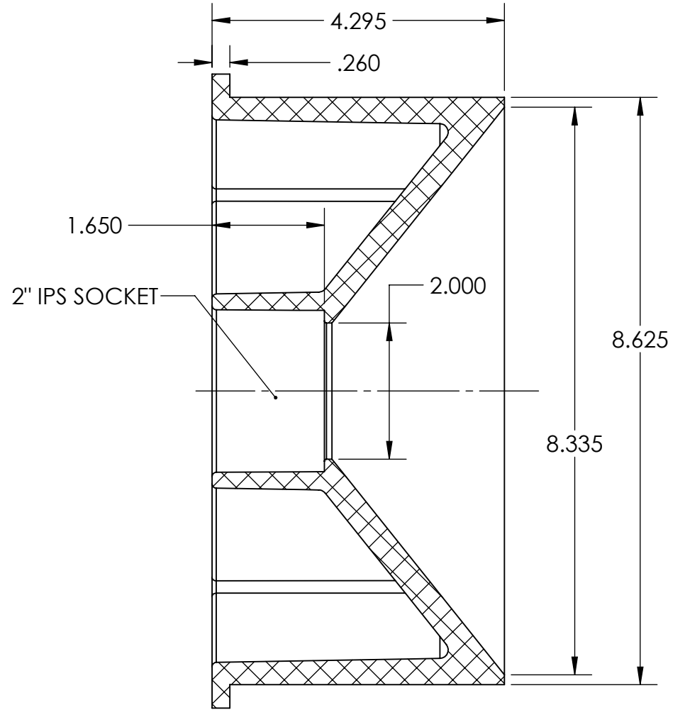
SECTION D-D SCALE 1 : 2
