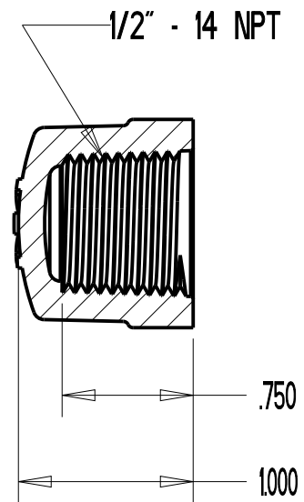
SECTION A-A SCALE 1.000
