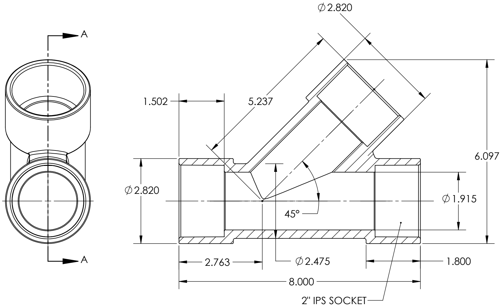
SECTION A-A
